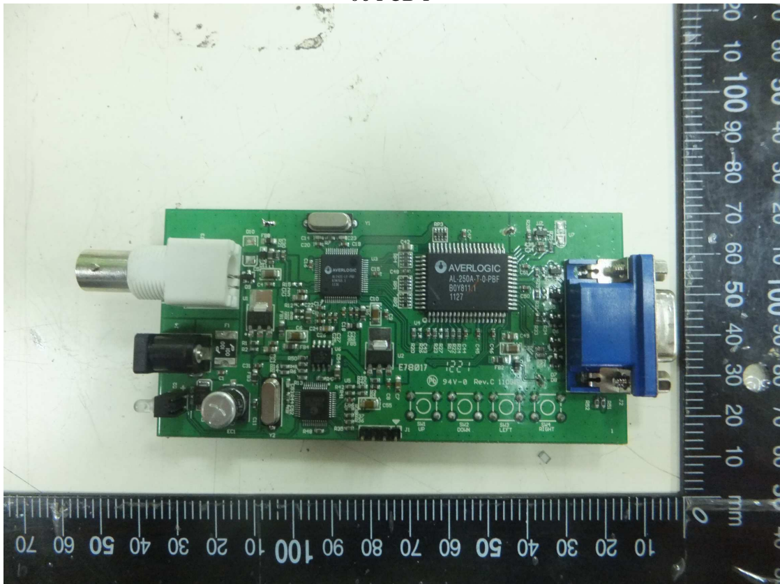
06 PCB-F
