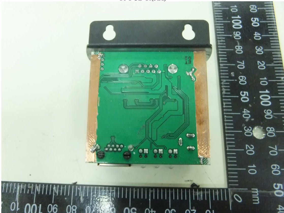
10 PCB-R(RX)
