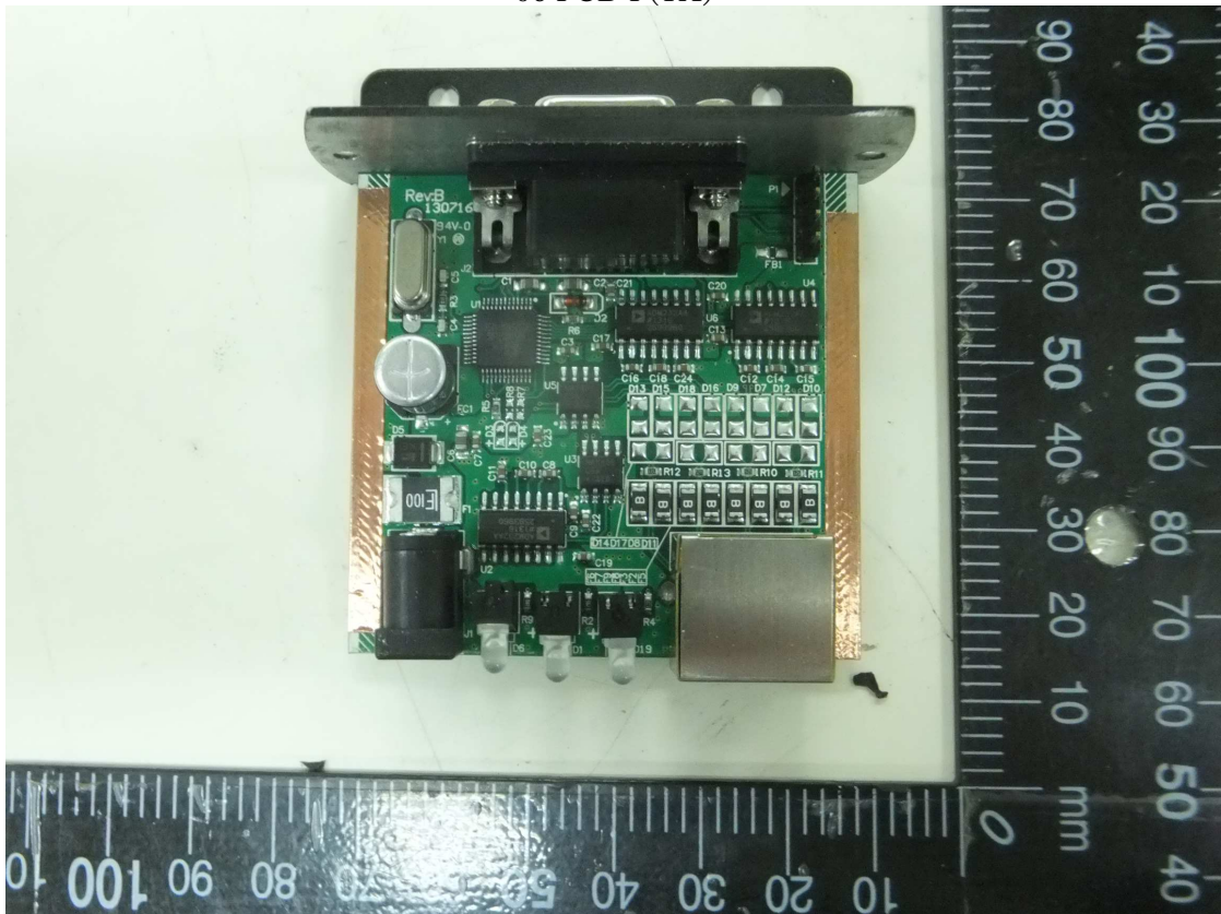
06 PCB-F(TX)
