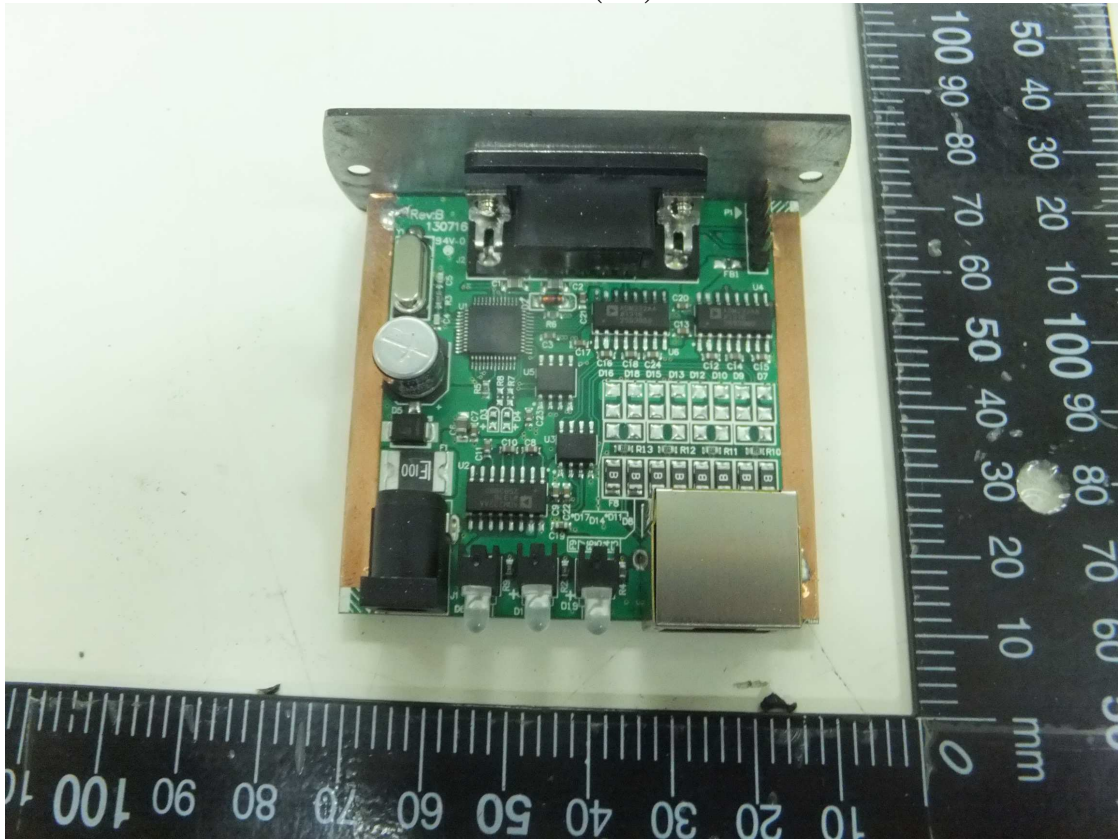
09 PCB-F(RX)
