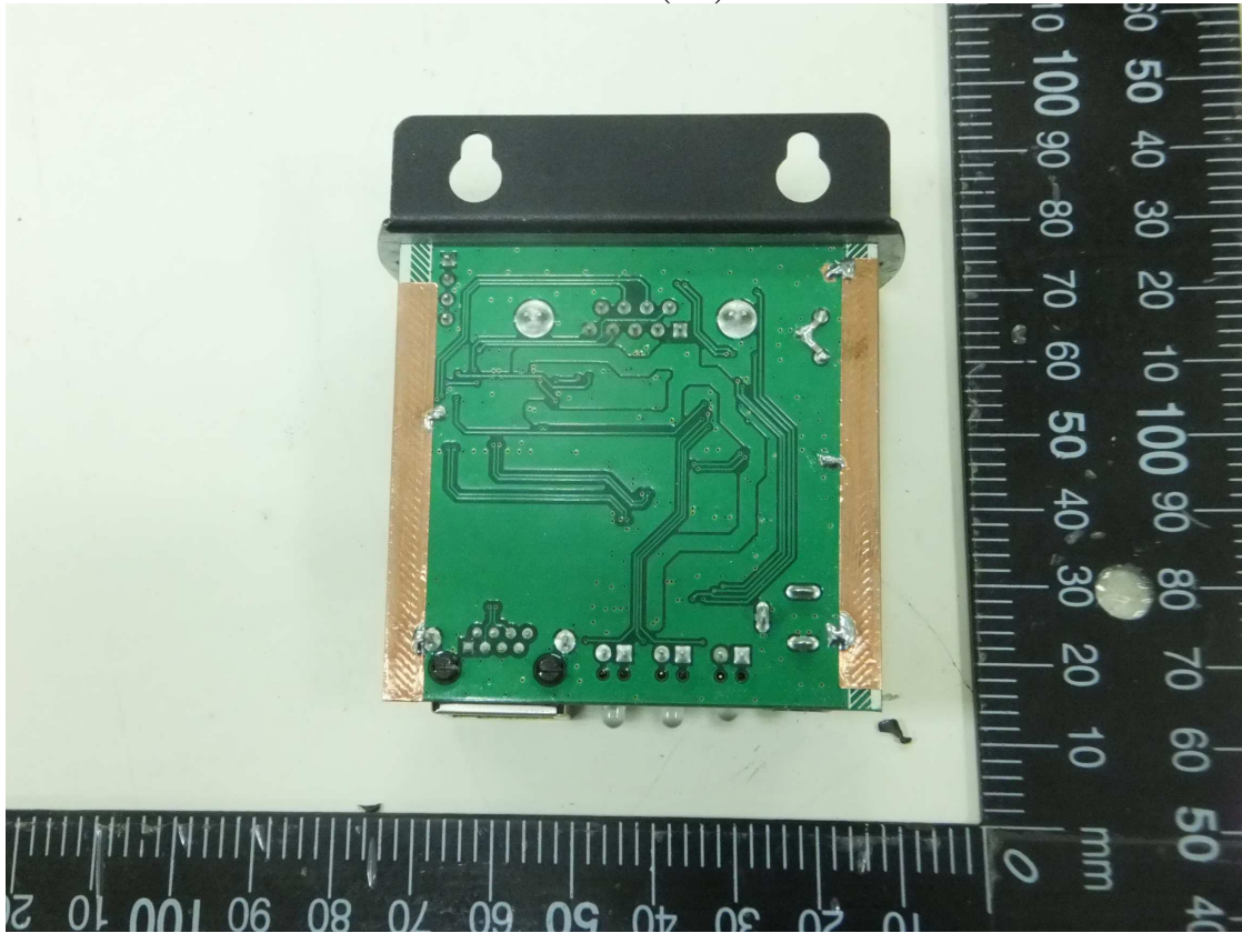
07 PCB-F(TX)
