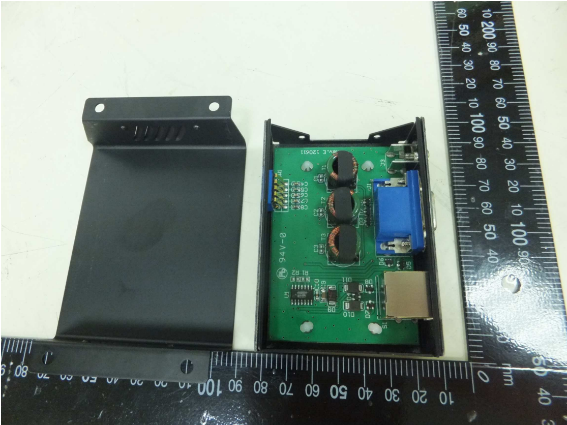
04 EUT 1 INSIDE
