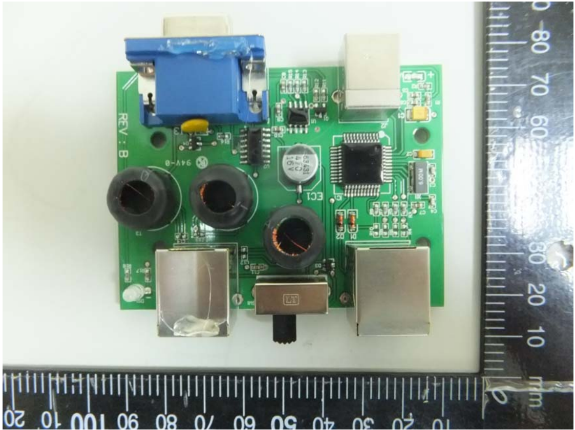
11 PCB-F
